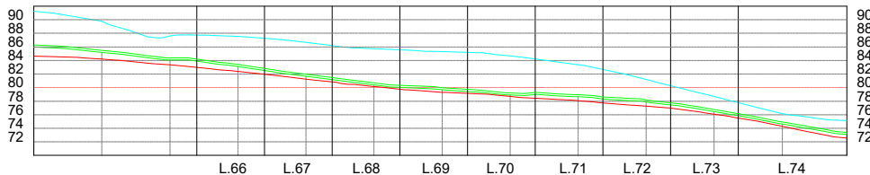
Perfil Longitudinal Q.197, L.66 à L.74
