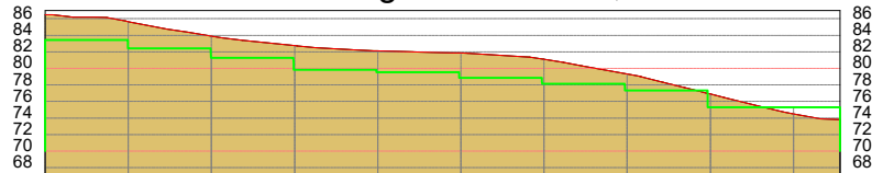
Perfil Longitudinal Q.197, meio
