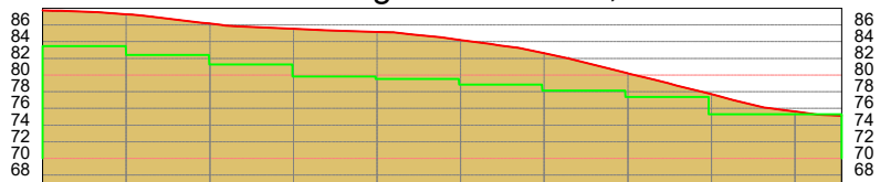
Perfil Longitudinal Q.197, fundos
