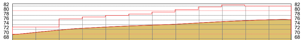
Perfil Longitudinal Q.182, fundos
