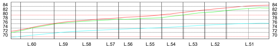
Perfil Longitudinal Q.182, L.51 à L.60, frente
